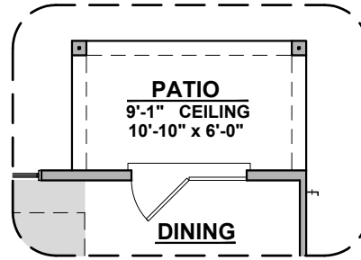
Center Hinge Door ILO Std. Door
