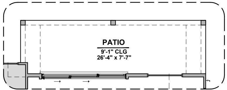
Stacking Door ILO STD. Door
