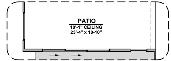
Stacking Door ILO Standard Door
